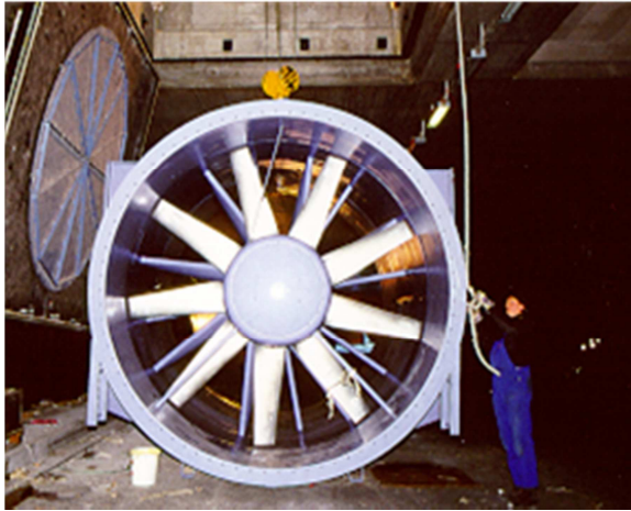
Installazione completa di un ventilatore assiale
