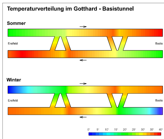
Simulazione del clima nella galleria del San Gottardo
