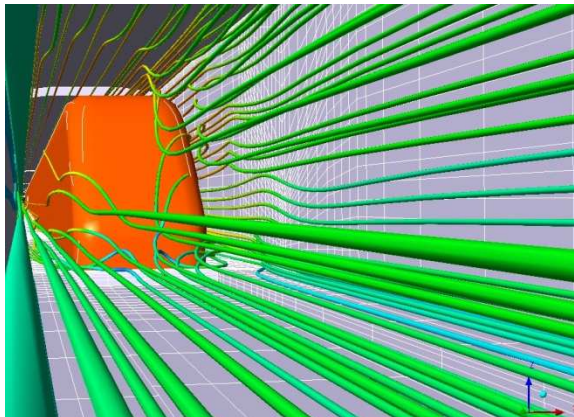
Visualizzazione del flusso d'aria in una galleria ferroviaria
