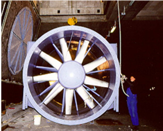
Installation complète d'un ventilateur
