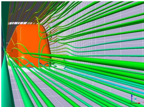
Visualisation des courants dans un tunnel ferroviaire
