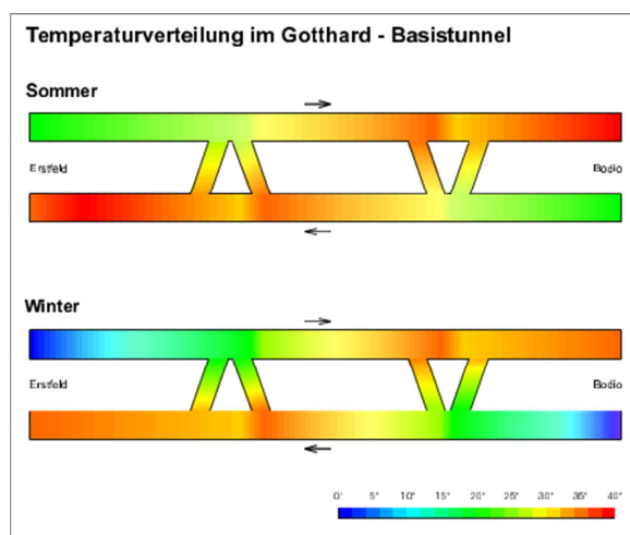
Calculs climatiques pour le tunnel de base du Gotthard
