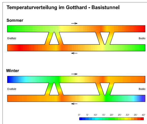
Klimaberechnung für den Gotthard – Basistunnel
