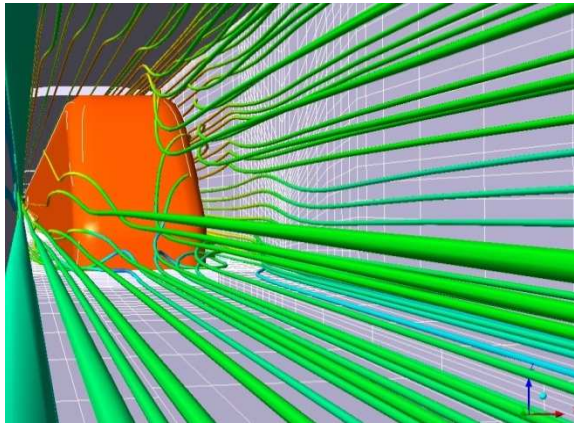
Visualisierung von Luftströmungen in einem Bahntunnel
