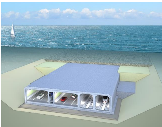
Sezione della galleria Fehmarn Belt, lungo 18 km (DE/DK)
