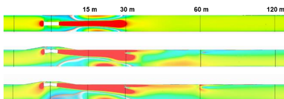
Calcoli CFD: configurazioni del ventilatore a getto
