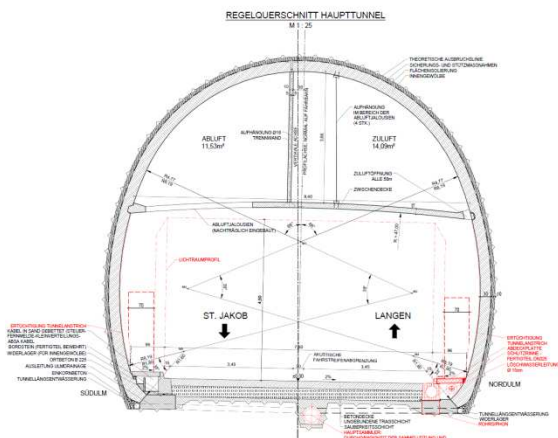
Sezione tipo della galleria esistente (le modifiche relative al 1. risanamento parziale sono in colore rosso)
