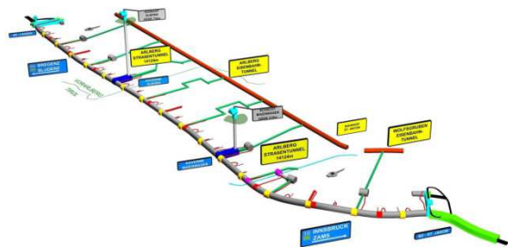
Rappresentazione schematica della galleria stradale dell'Arlberg, tra l'altro con le seguenti variazioni previste: entrate e uscite verso e dal canale di immissione aria (AZ) a distanza di <500 m nonché 8 piazzole di emergenza aggiuntive sul lato nord
