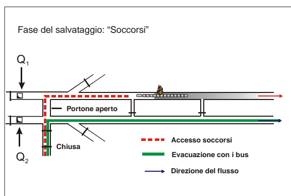
Concetto di fuga e salvataggio per una galleria ferroviaria
