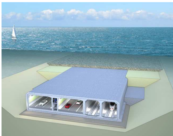
Sektion des 18 km Fehmarnbelttunnels (DE/DK)
