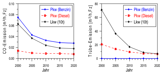
Basiswerte der Kohlenmonoxid-Emission und Sichttrübe (RABT-2006)
