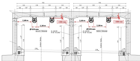
Anordnung der Strahlventilatoren in den Decken-nischen
