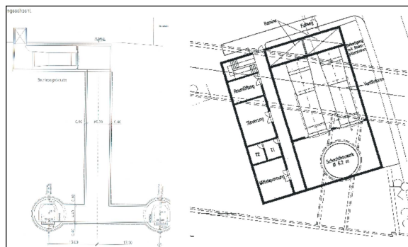
Längsschnitt und Grundriss eines Entrauchungsschachtes des Feuerbacher Tunnels
